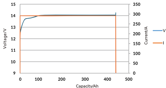
12V460Ah 300A charge @RT
